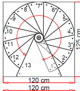
13 Stufen (Standard+1 Höhererw.) 13 steps (standard+1 height extension)
