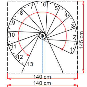
13 Stufen (Standard+1 Höhererw.) 13 steps (standard+1 height extension)
